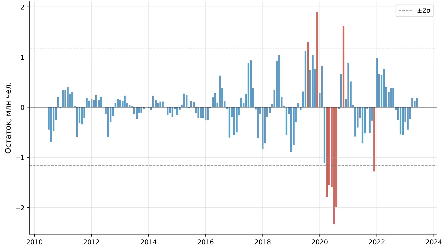
Остаточная компонента декомпозиции
