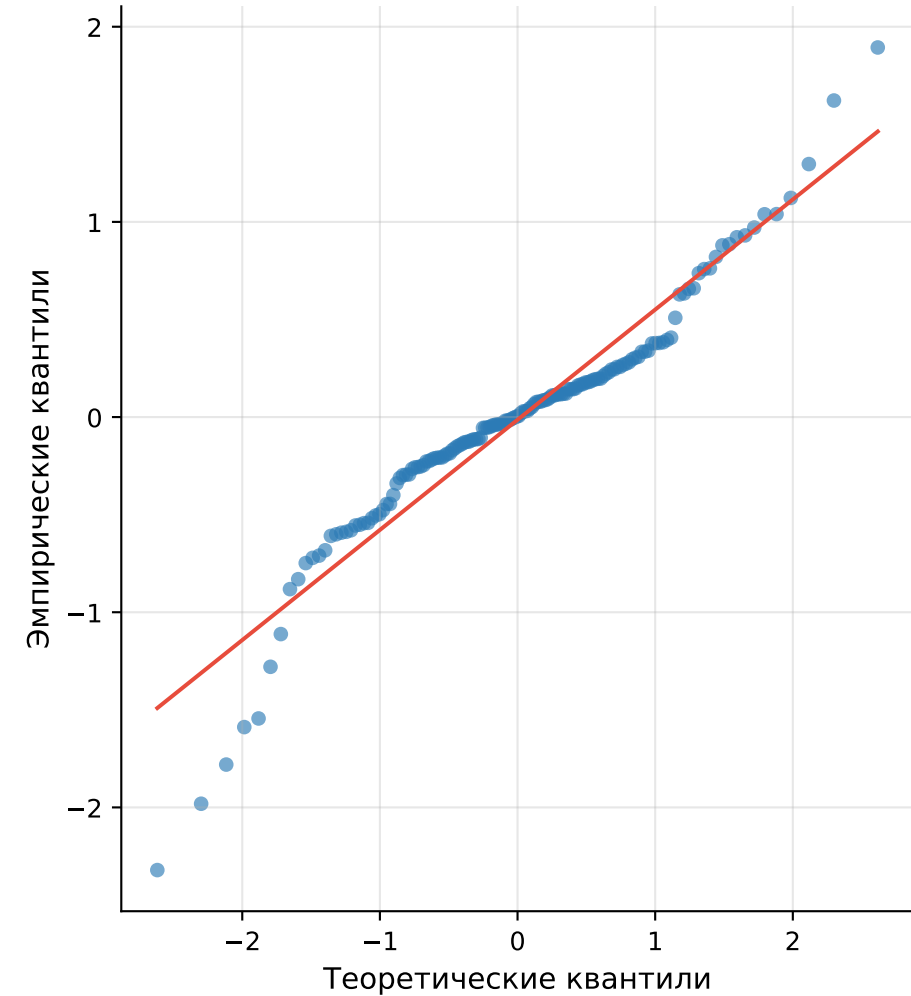
Q-Q нормальности остатков
