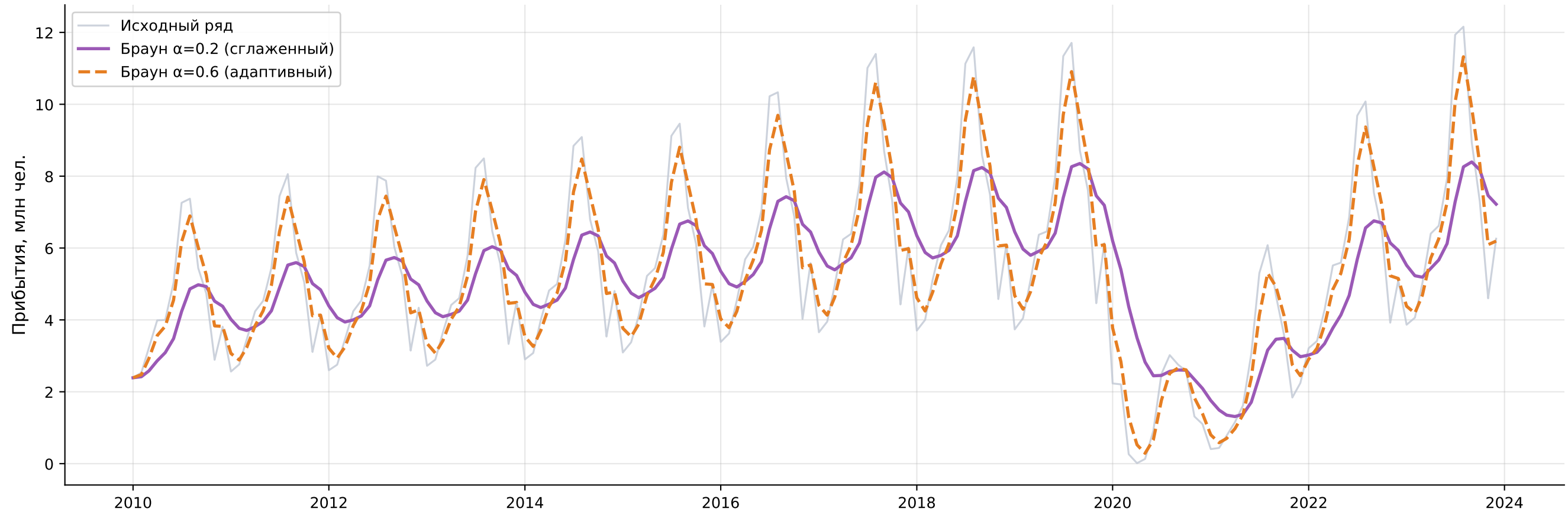
Экспоненциальное сглаживание Брауна: \alpha=0.2 и \alpha=0.6
