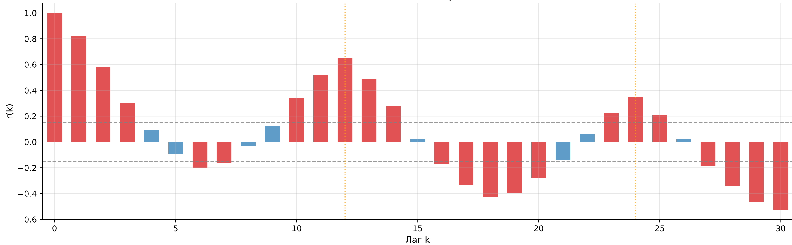
(а) Исходный ряд
