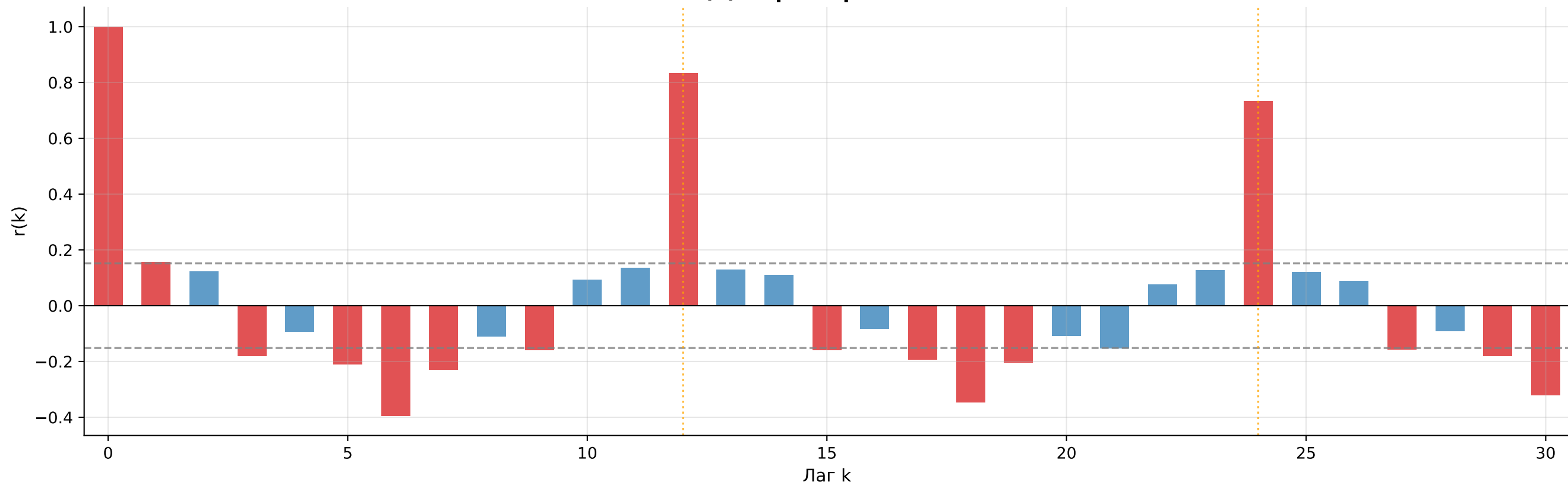
(б) Первые разности
