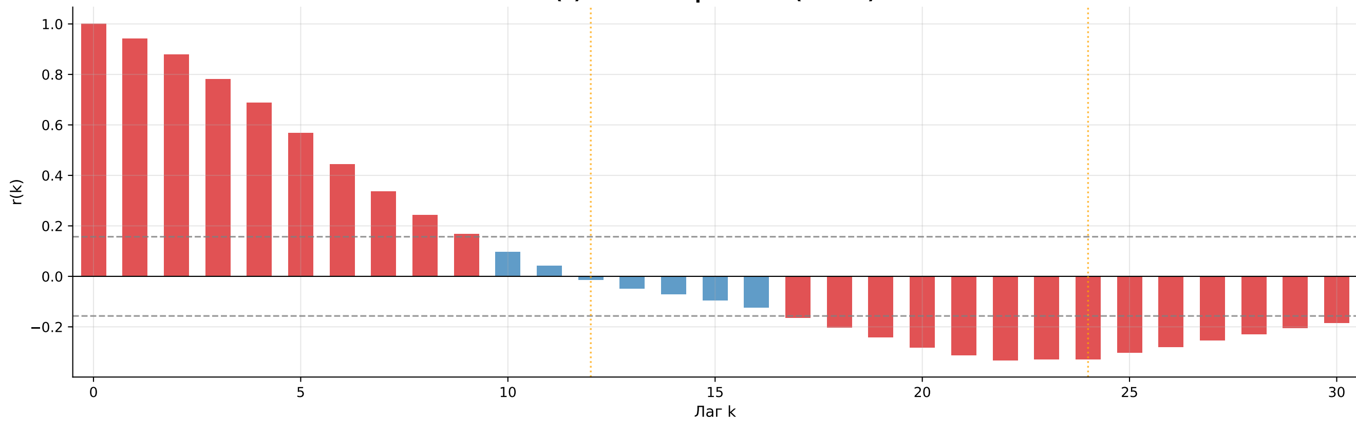
(в) Сезонные разности (лаг 12)
