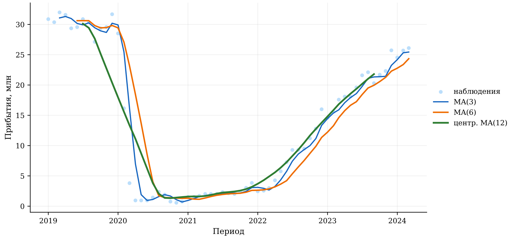
Сглаживание ряда скользящими средними различной ширины
