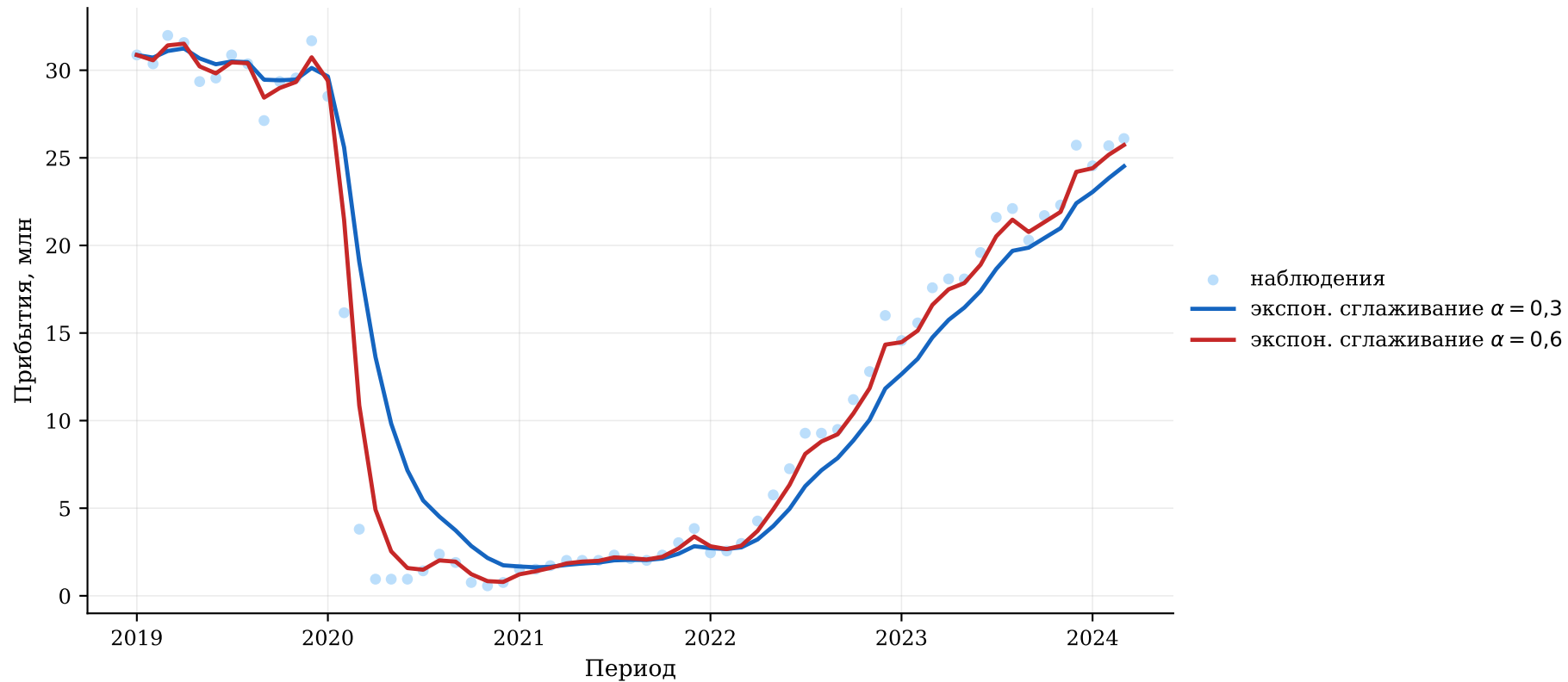
Экспоненциальное сглаживание Брауна при двух значениях параметра \alpha
