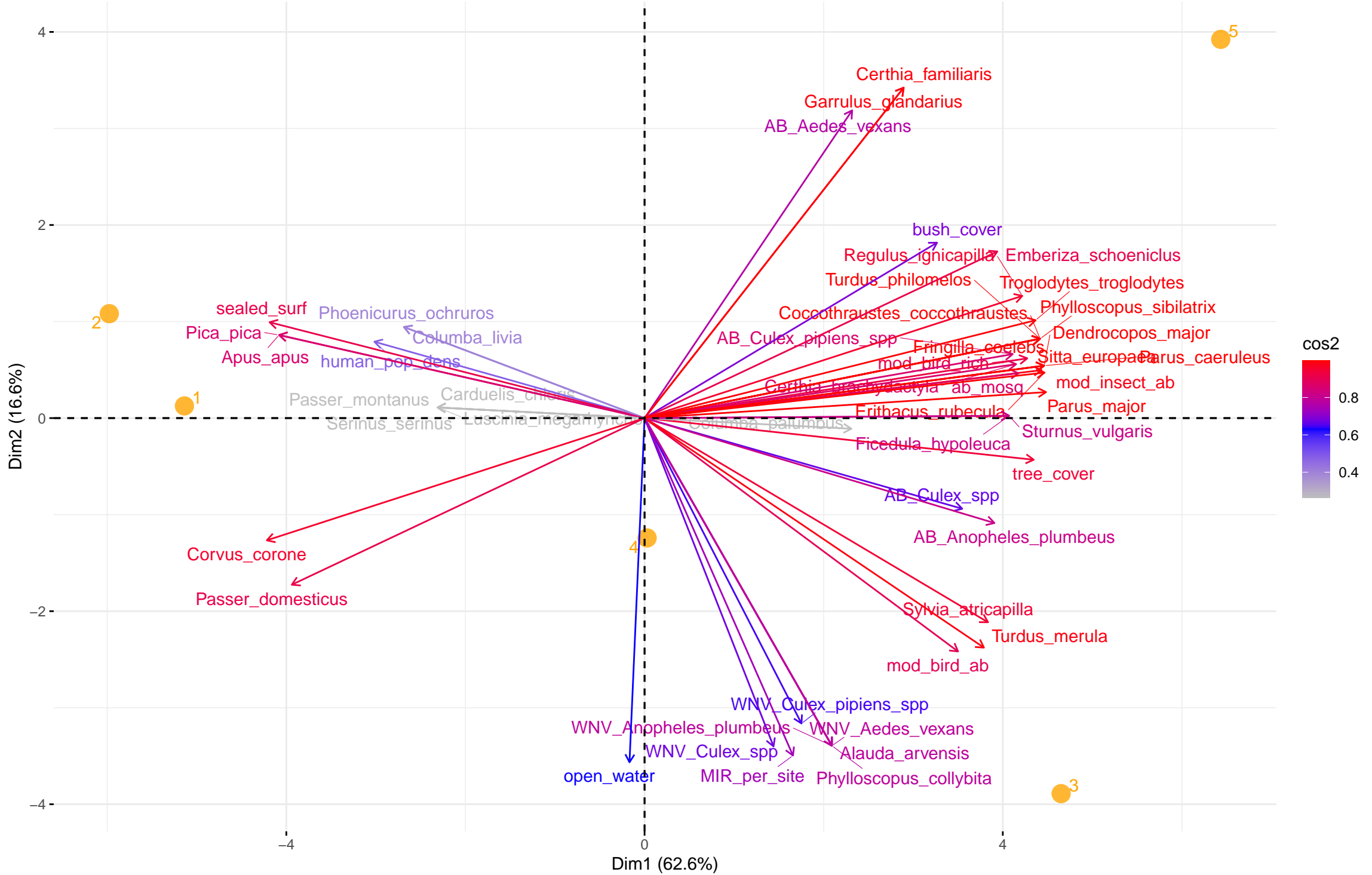
PCA – Biplot
