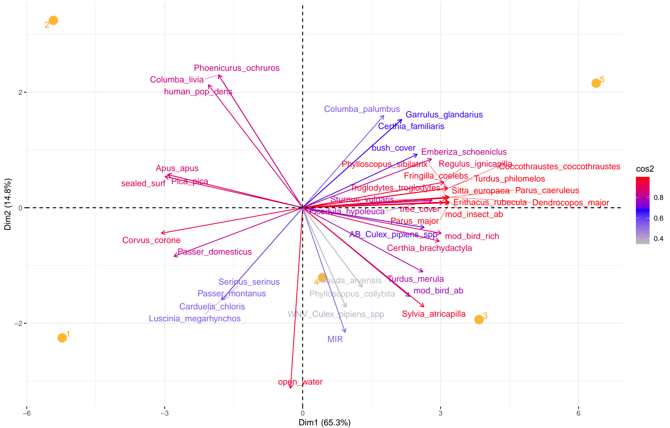
PCA – Biplot
