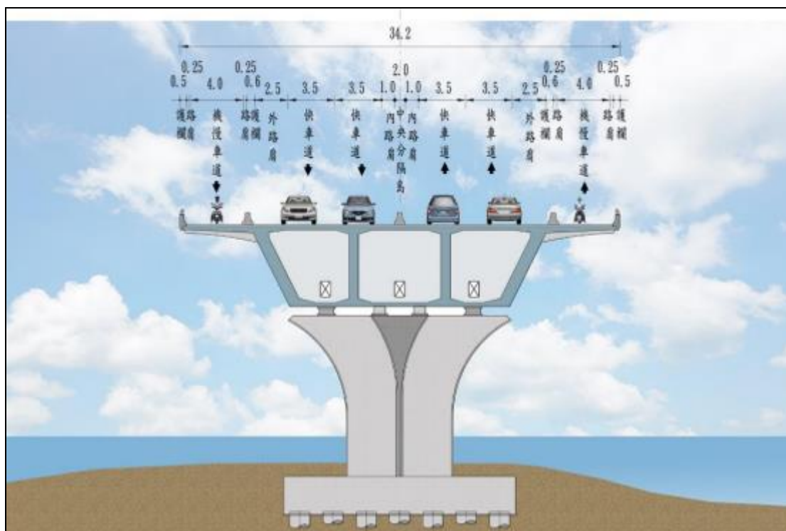
圖 6-4 主橋段標準斷面圖
