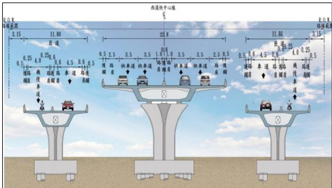
圖 6-2 主橋段脊背橋模擬圖
