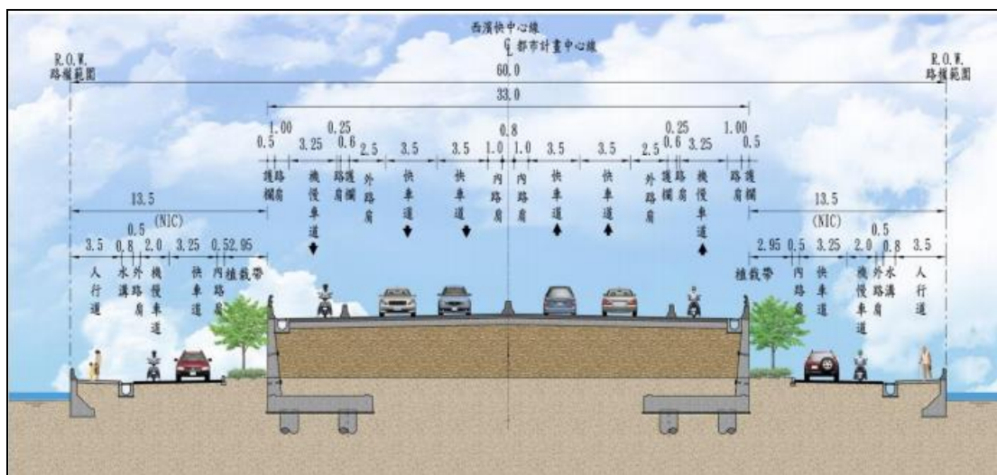
圖 6-5 終點段標準斷面圖
