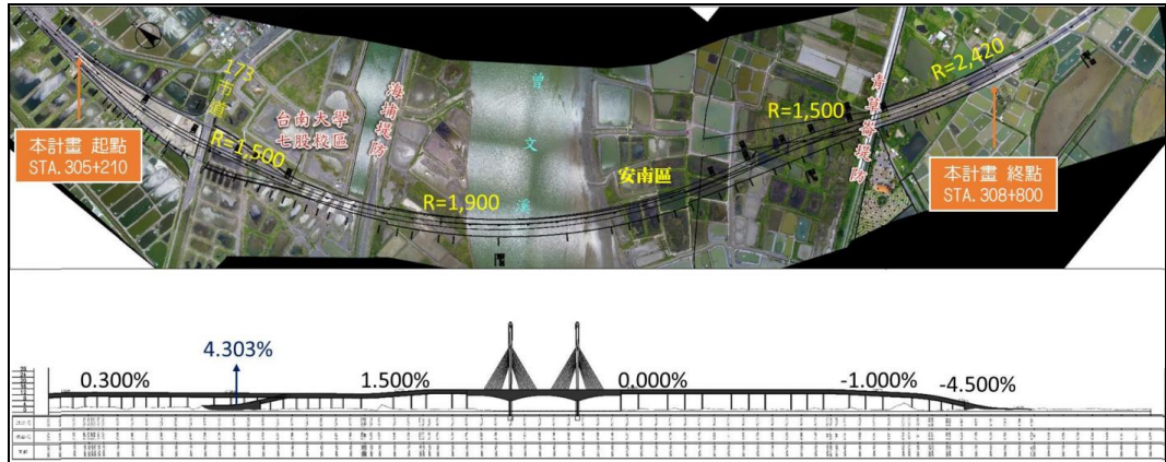
圖 6-1 本案道路平、縱面圖
