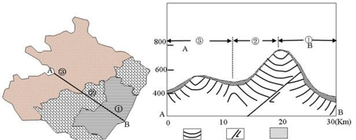
图 1 华北某山区泥石流危险性区划示意图
