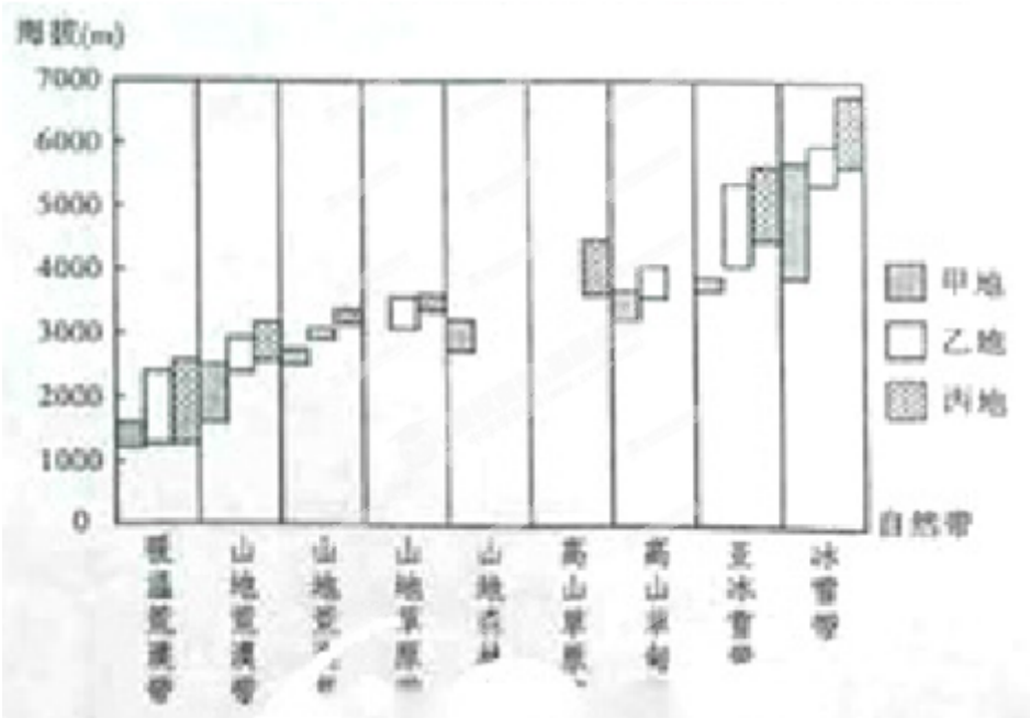
图 4 为我国某山地北坡甲、乙、丙三地垂直自然带随海拔变化示意图。完成下列各题。
