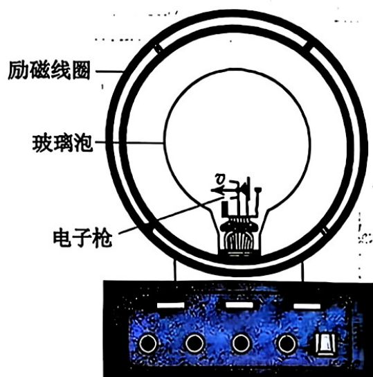
图甲 洛伦兹力演示仪示意图
