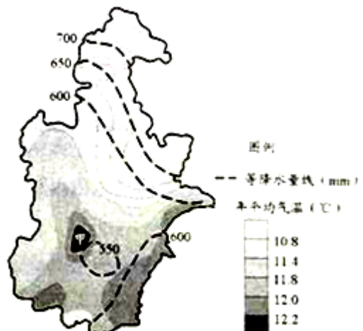
图 2 天津市年平均气温和降水分布图
