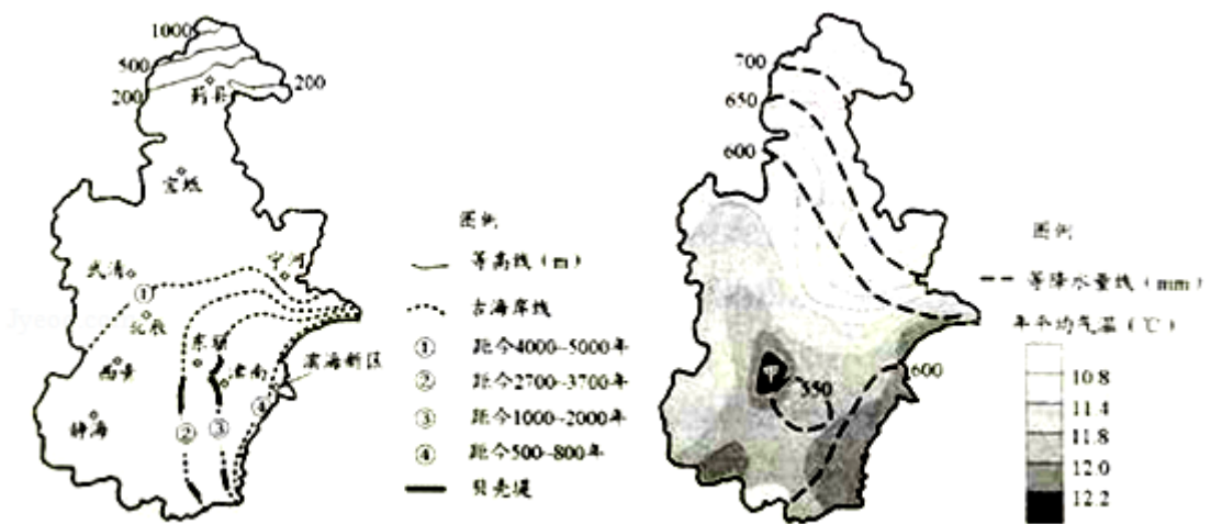
图 1 天津市等高线和古海岸线分布图
