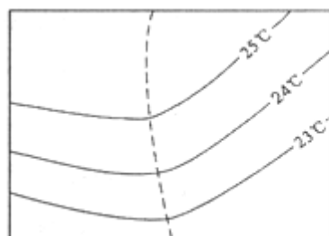
图1 某海域8月表层水温分布图
