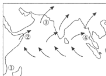
图2 北印度洋夏季季风示意图
