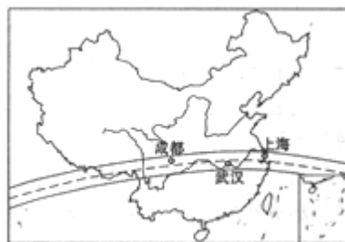
2009年7月22日月球本影扫过范围示意图
