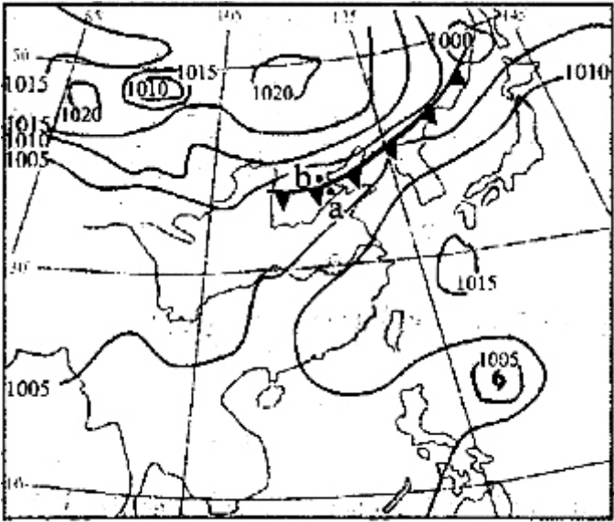
图 6（符号 6 表示台风）
