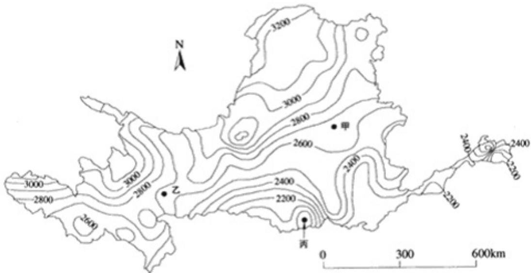
图4 黄河流域多年平均年有效辐射总量等值线图（单位：MJ/m 2 ）
