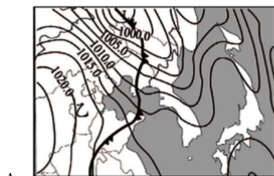
乙地某次浮尘天气形成过程示意图
