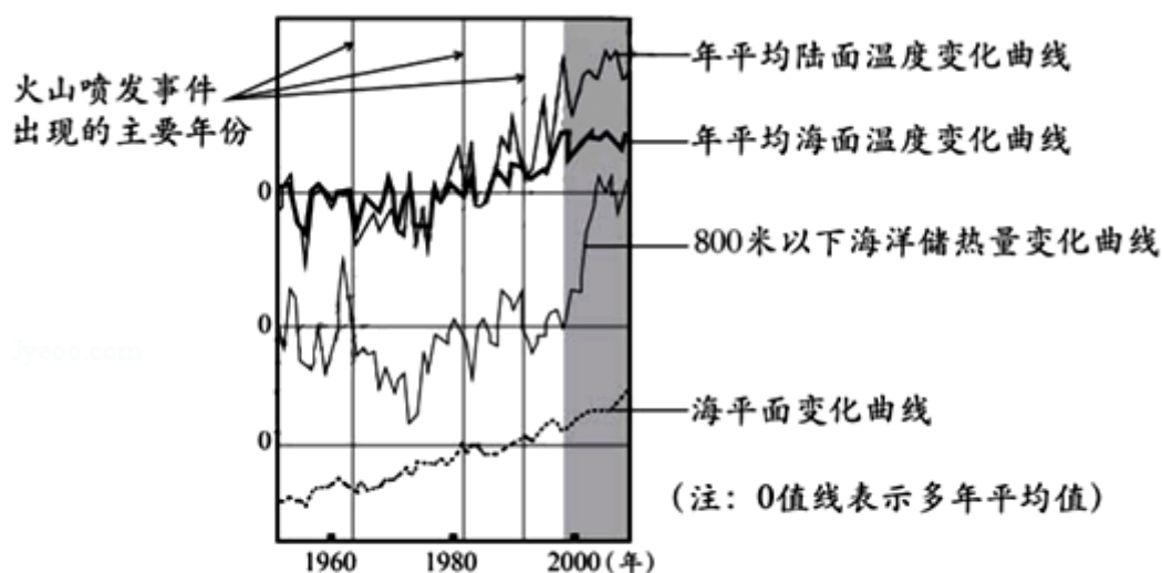
全球变暖相关数据变化趋势示意图
