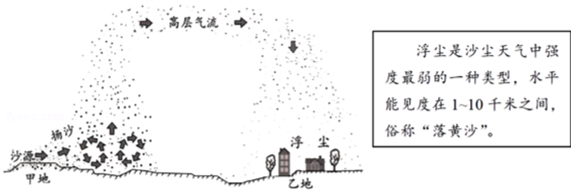
乙地某次浮尘天气形成过程示意图
