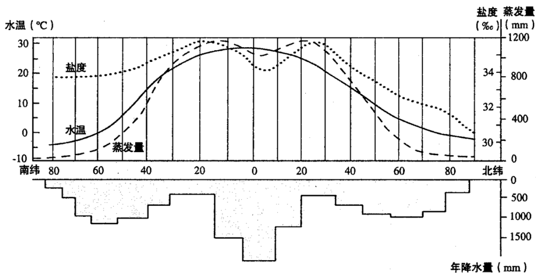
全球年降水量及海洋表面平均温度、蒸发量与盐度按纬度的分布
