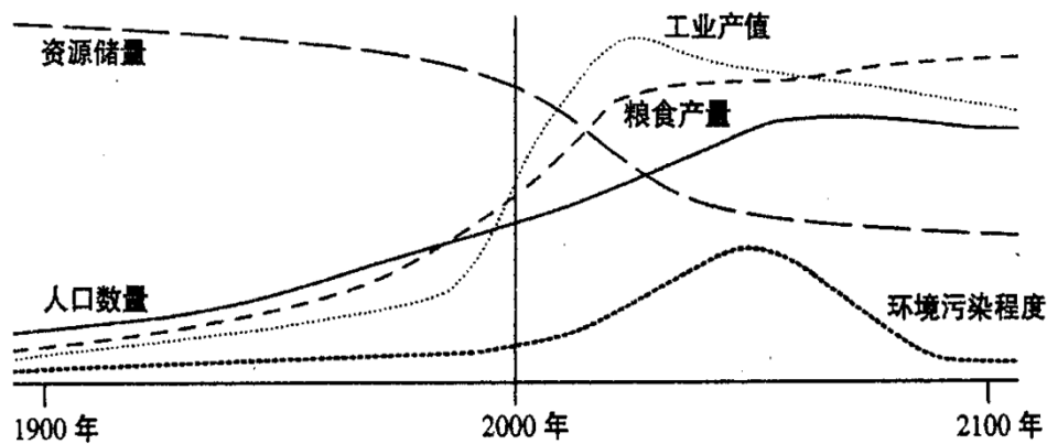
图2 人口数量变化与环境诸要素相互关系模式
