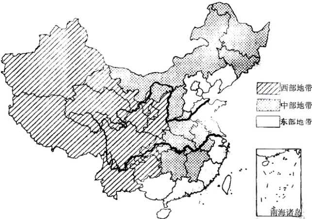
图 19 中国三大经济地带分布图
