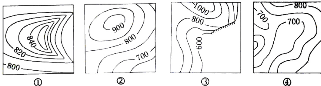
图2 等高线示意图
