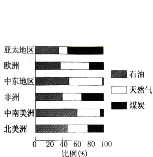
图11 世界各地区化石能源消费结构图（2006年）
