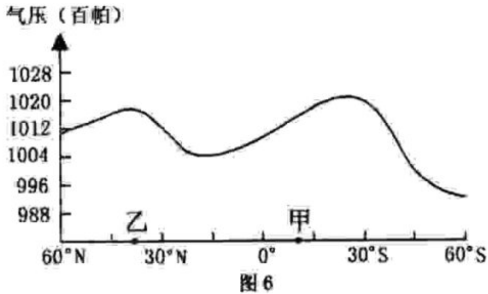
图6为“某月沿0°经线海平面平均气压分布图。
