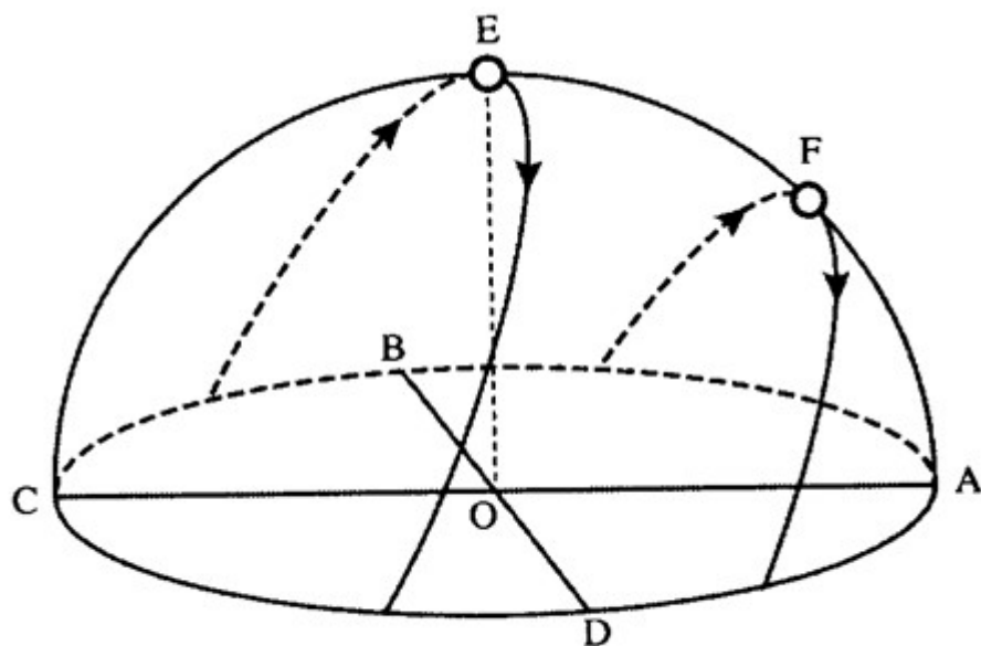
某地二至日太阳视运动轨迹示意图
