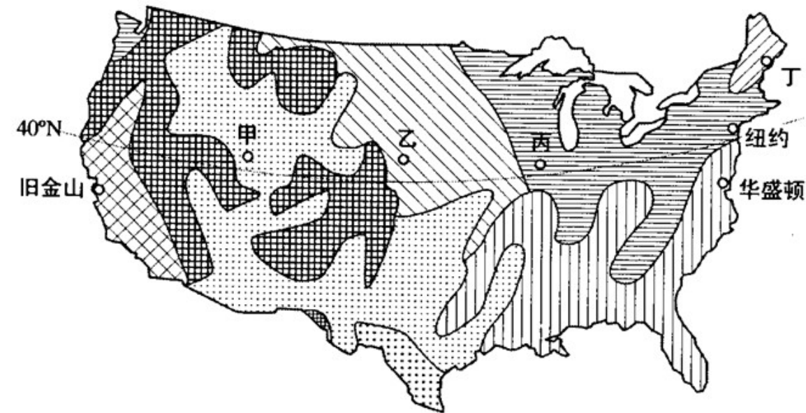
美国本土自然带分布示意图
