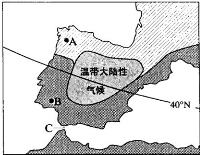
伊比利亚半岛气候示意图
