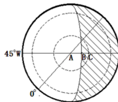
地球晨昏线示意图
