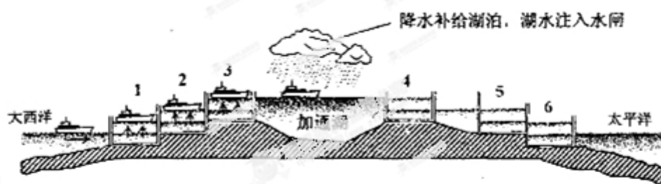
图 9 巴拿马运河通航原理示意图
