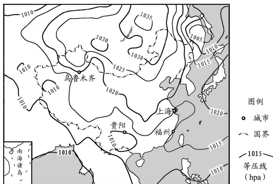
图 5 某日 14 时海平面气压场分布图
