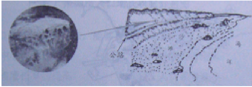
图2 古海蚀地貌位置示意图
