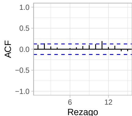
FAC residuos^2 ARMA
