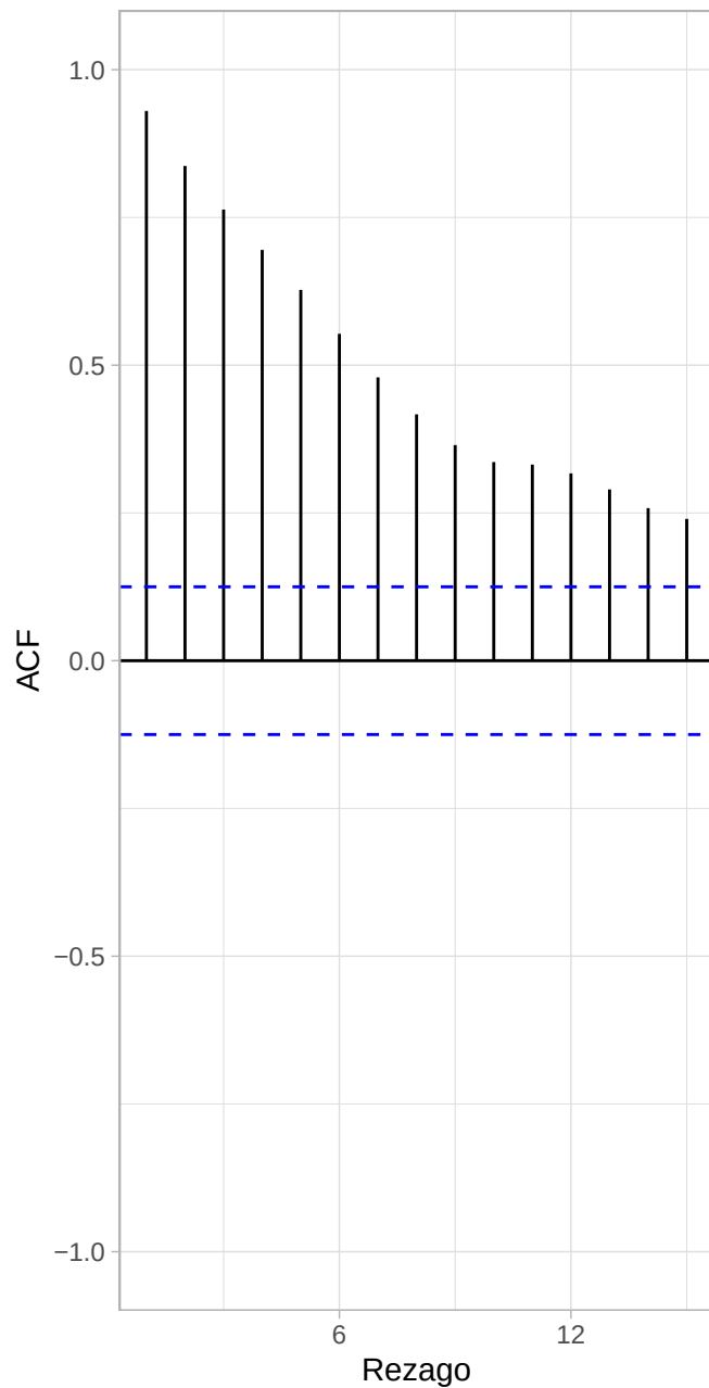
FAC del logaritmo precio del te
