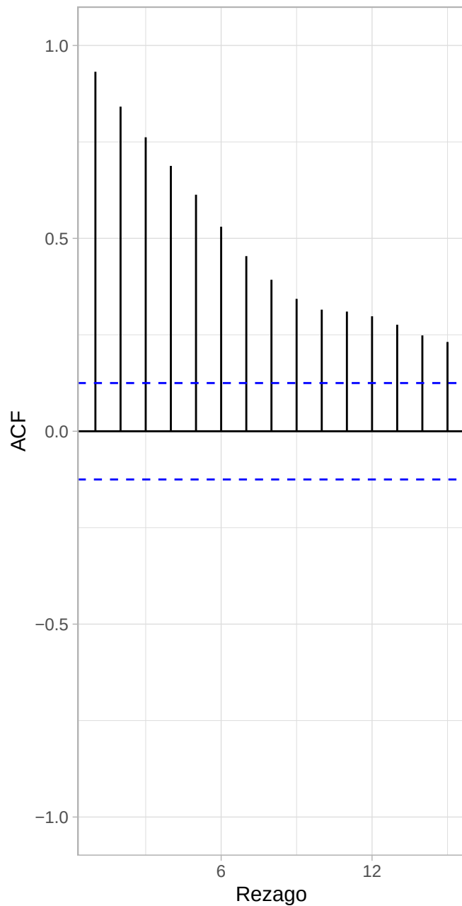
FAC del precio del te
