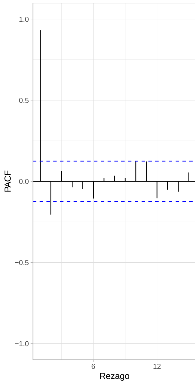
FACP del precio del te
