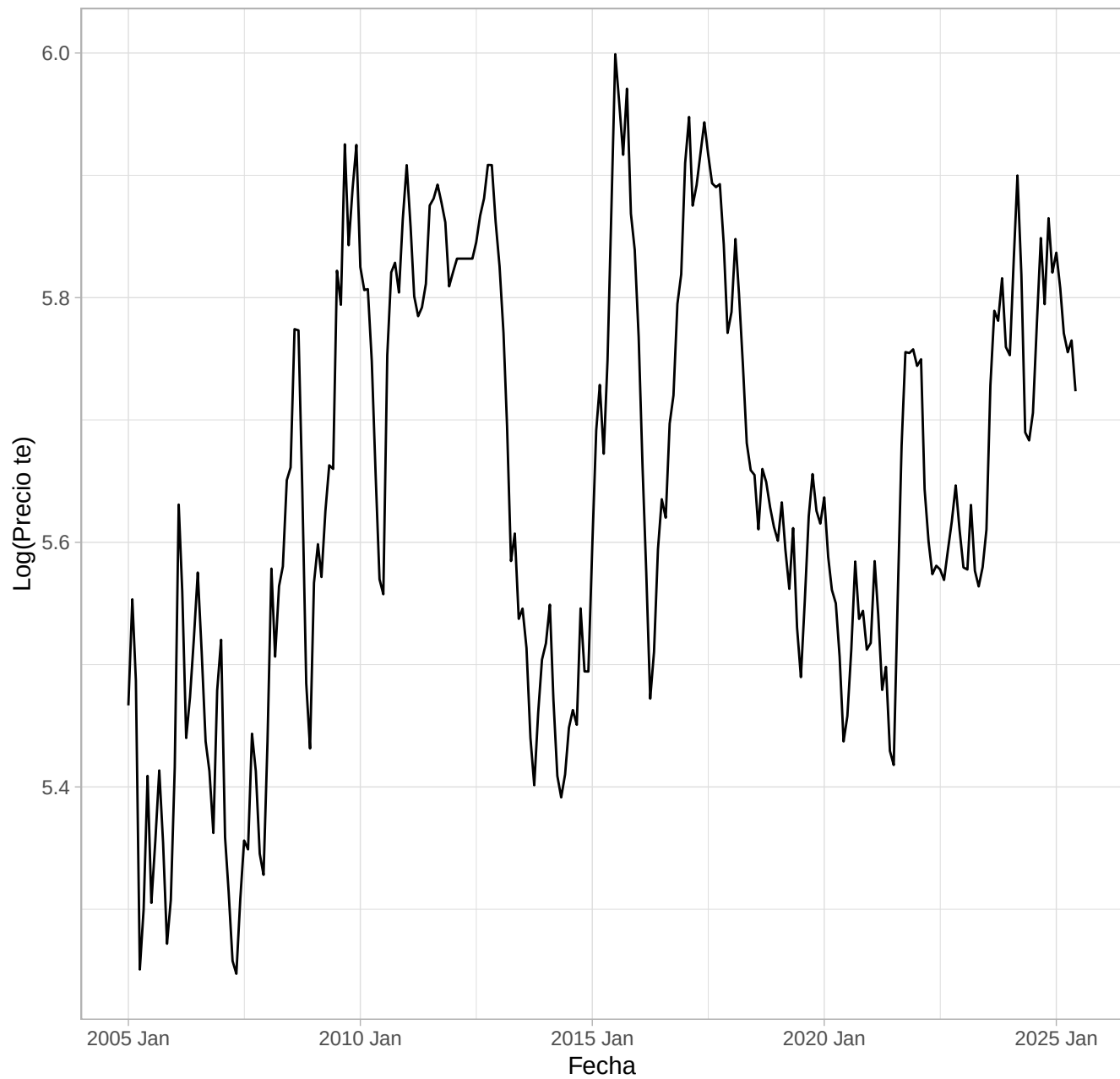
Logaritmo del precio internacional del te
