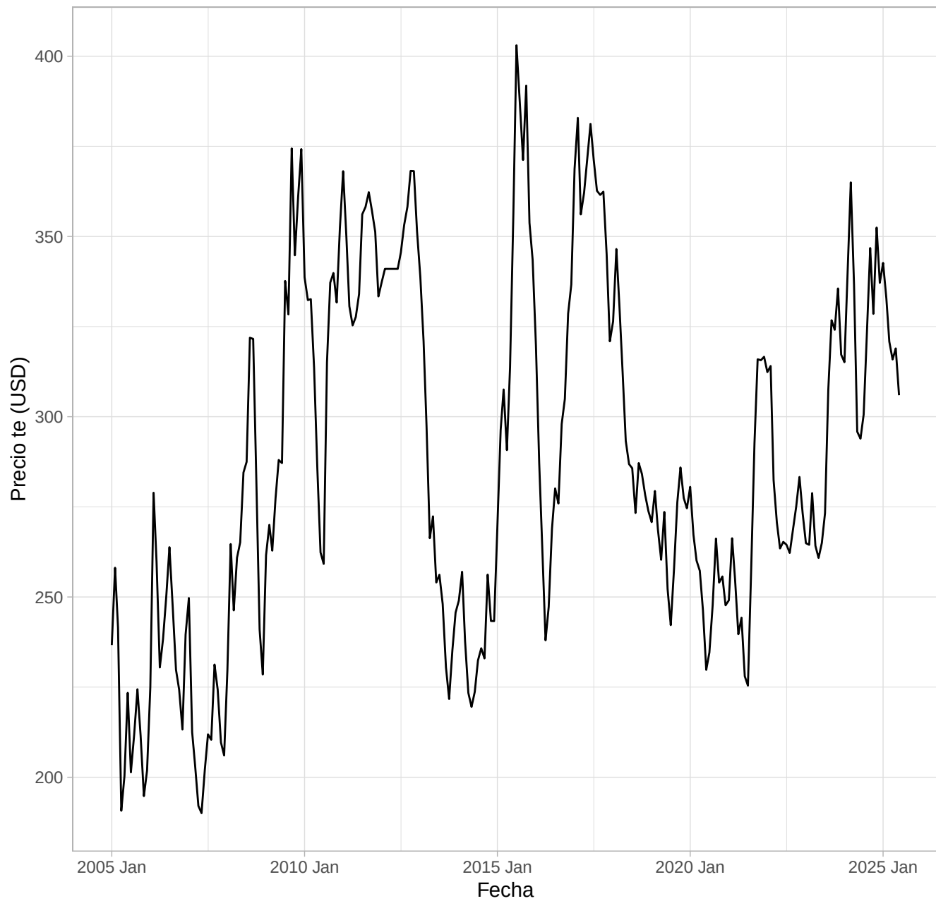
Precio internacional del te, 2005–2025
