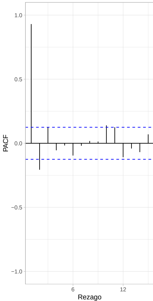
FACP del logaritmo precio del te
