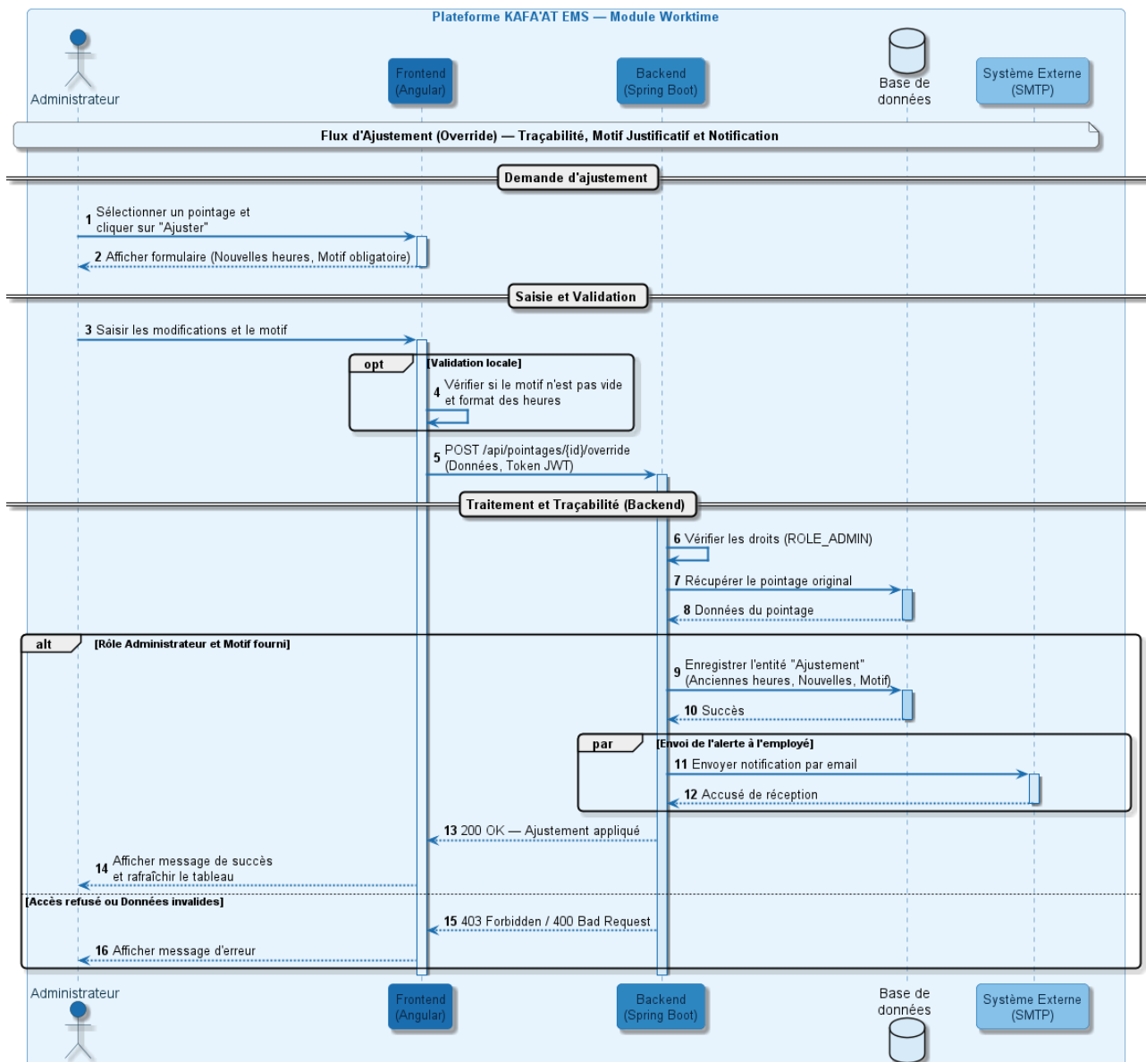
FIGURE 2.13 – Diagramme de séquence d'un ajustement de pointage (Override)
