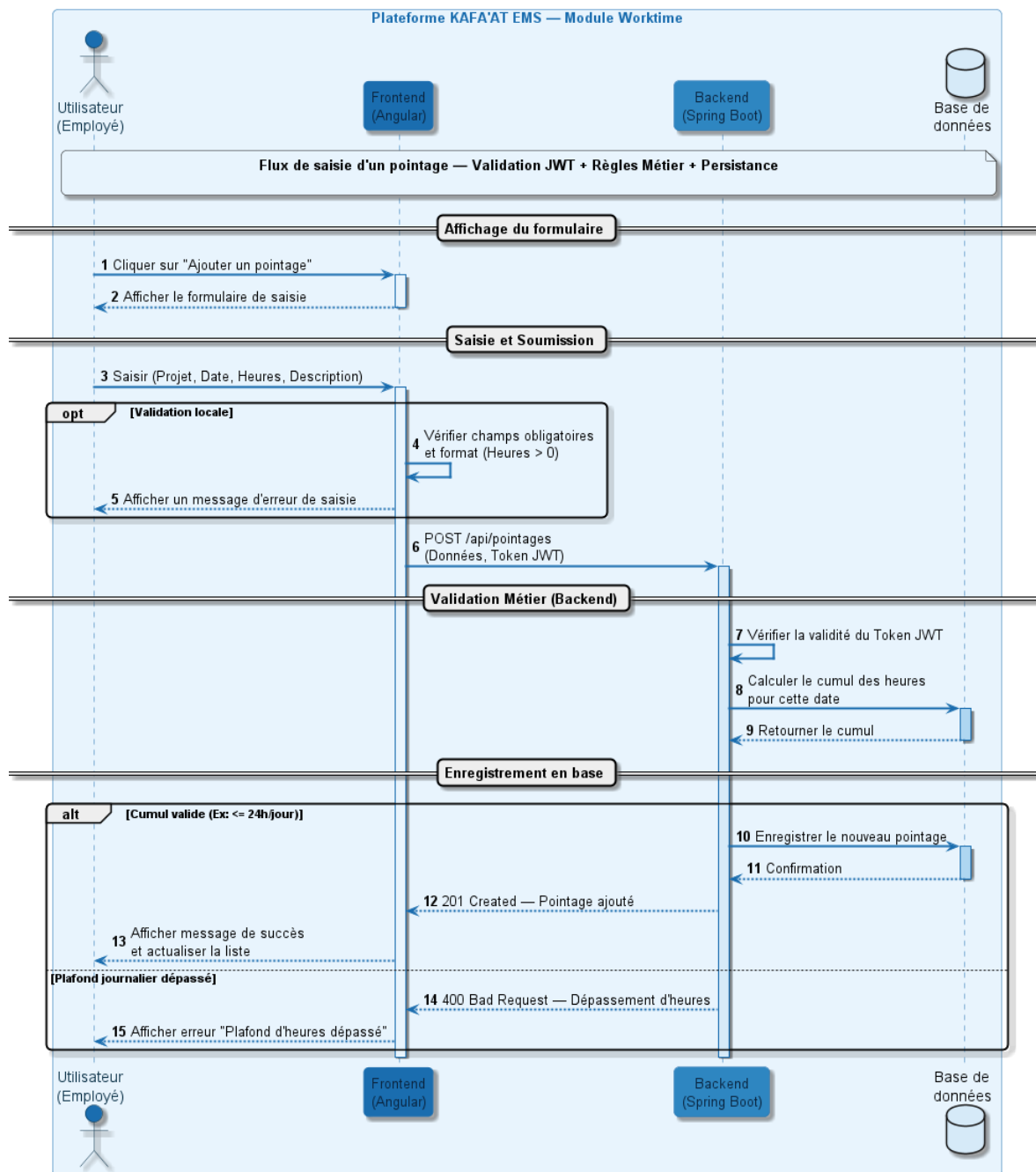
FIGURE 2.9 – Diagramme de séquence de la soumission d'un pointage
