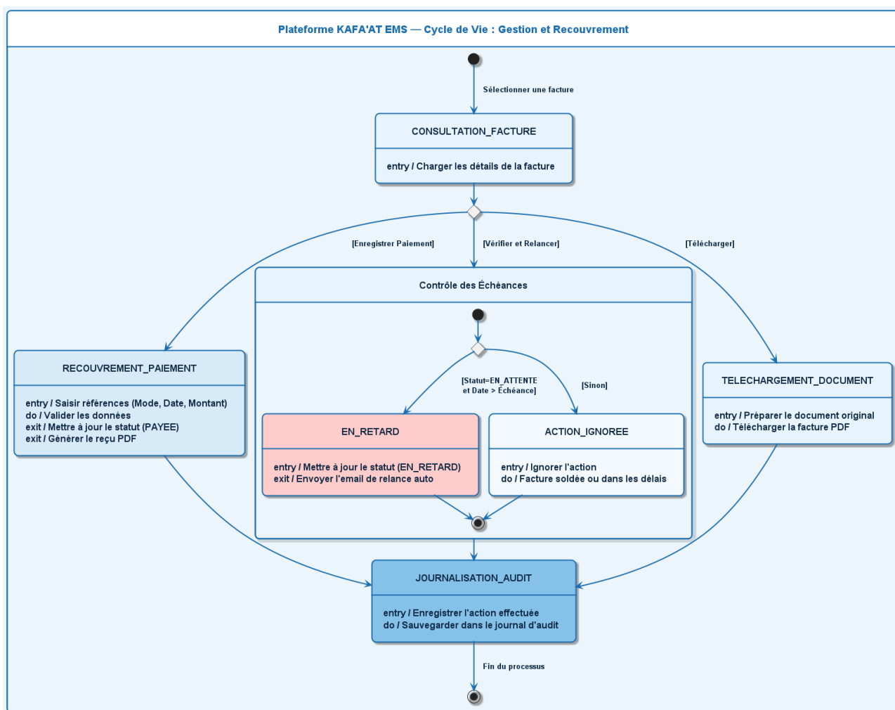
FIGURE 2.17 – Diagramme d'état-transition : Gestion, relances et recouvrement des factures
