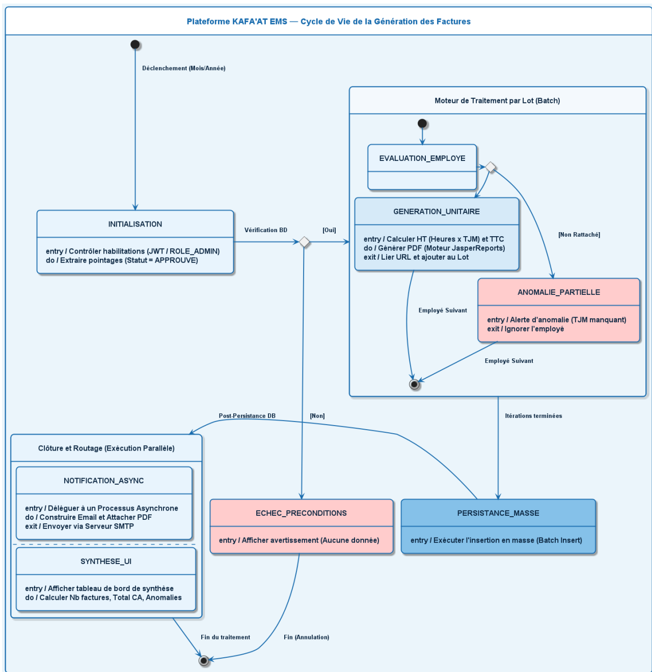
FIGURE 2.16 – Diagramme d'état-transition : Cycle de vie de la génération massive des factures
