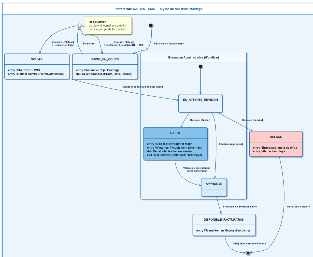
FIGURE 2.15 – Diagramme d'état-transition : Cycle de vie et validation d'un pointage
