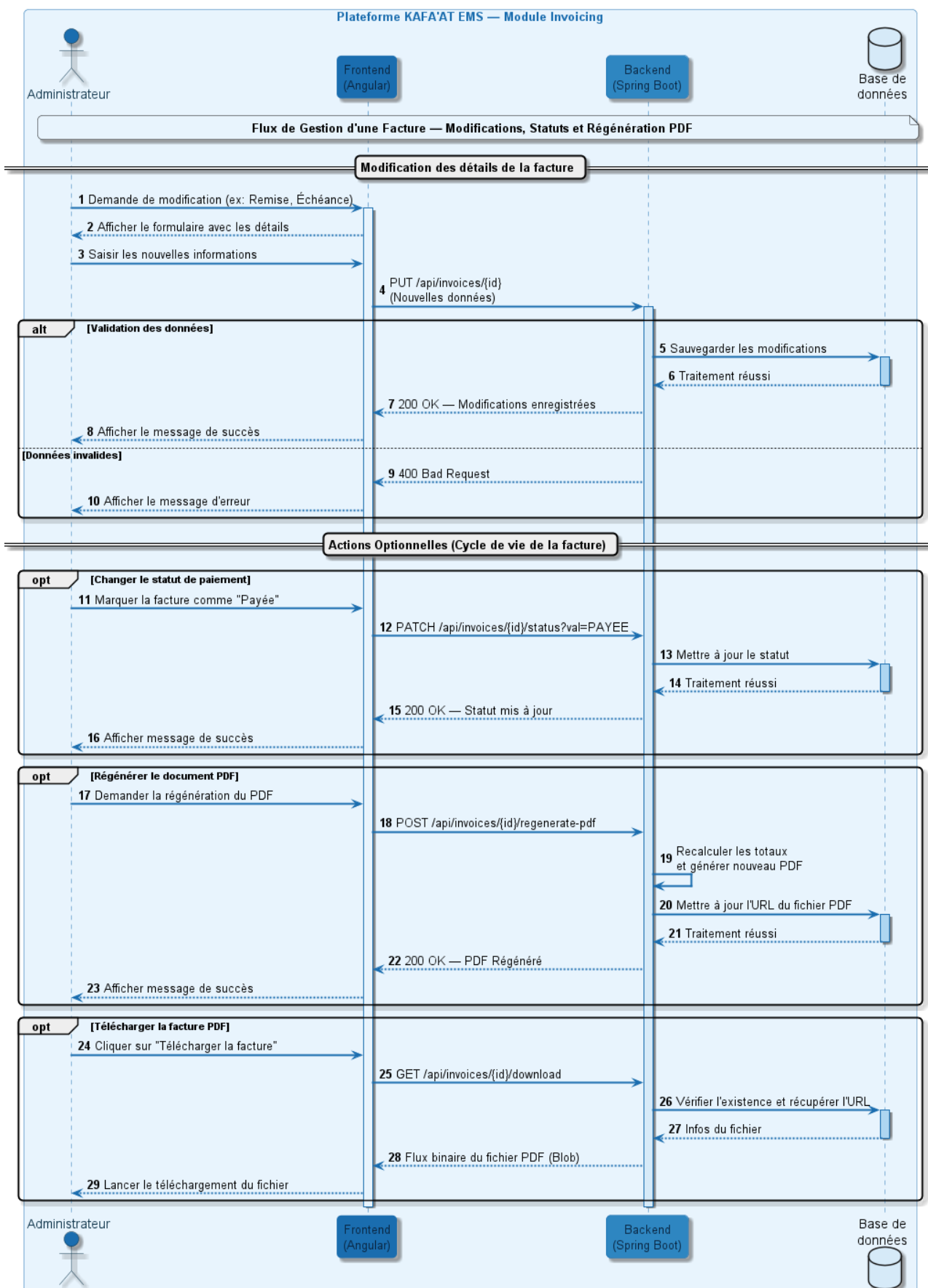
FIGURE 2.14 – Diagramme de séquence de la gestion détaillée d'une facture
