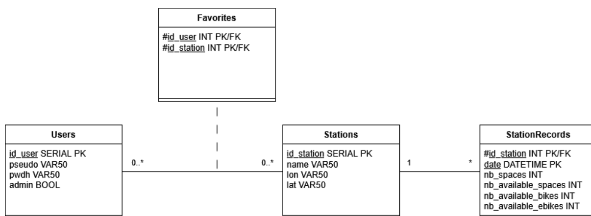
Figure 4: Diagramme UML du modèle de données
