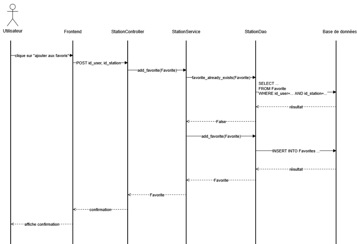
Figure 7: Diagramme de séquence de la fonctionnalité “ajouter une station favorite”
