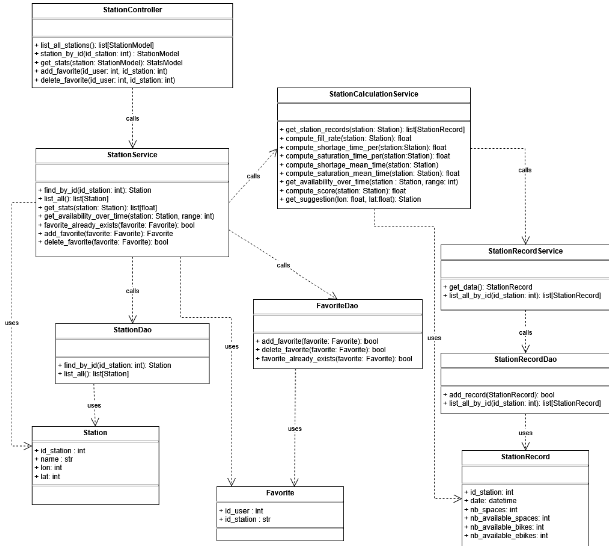
Figure 6: Diagramme de classes lié aux stations
