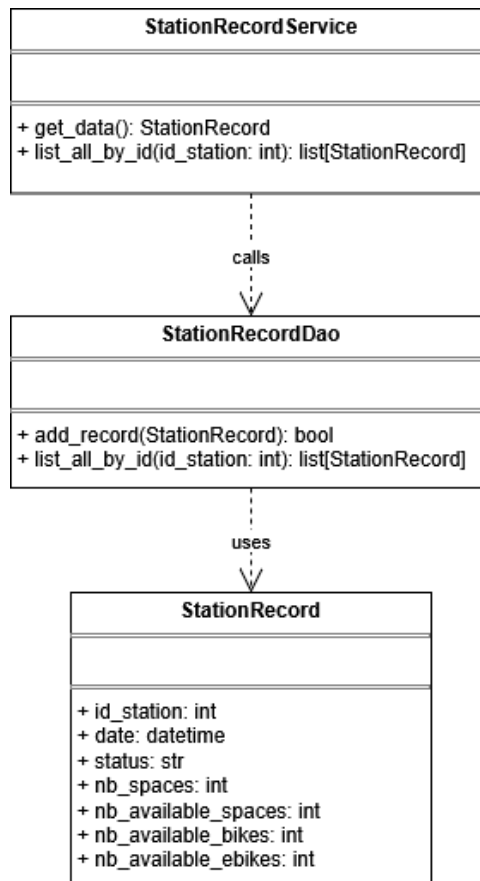
Figure 7: Diagramme de classes lié aux enregistrements
