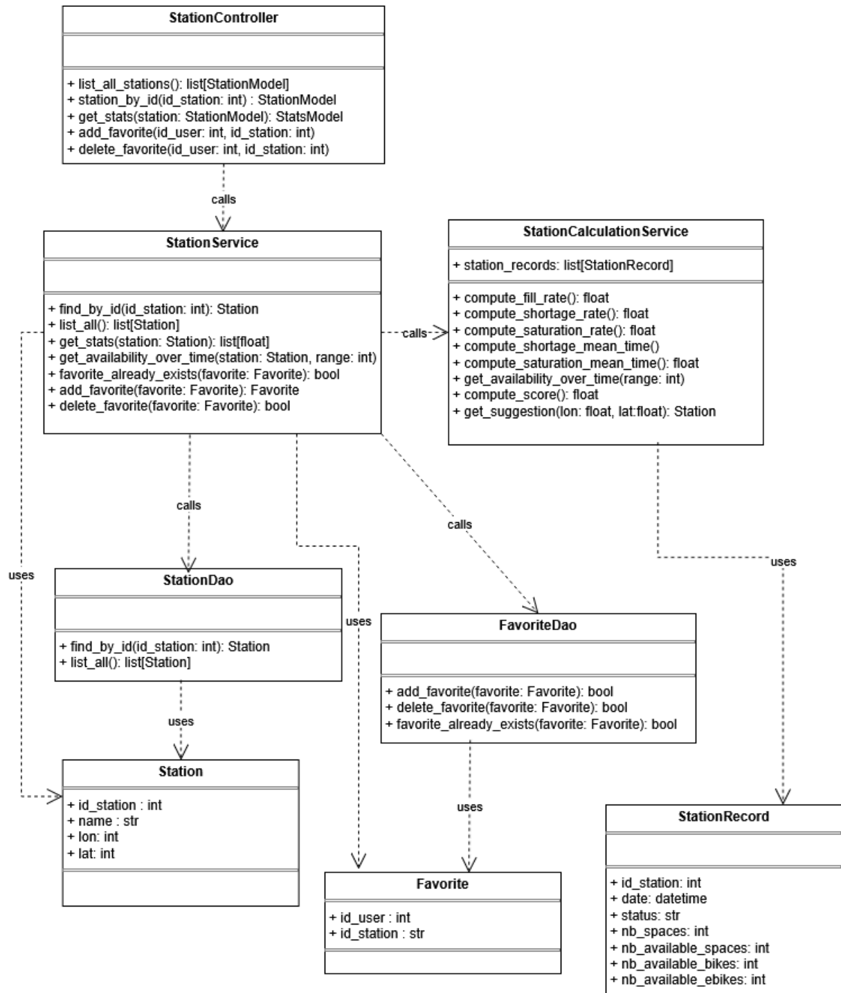
Figure 6: Diagramme de classes lié aux stations
