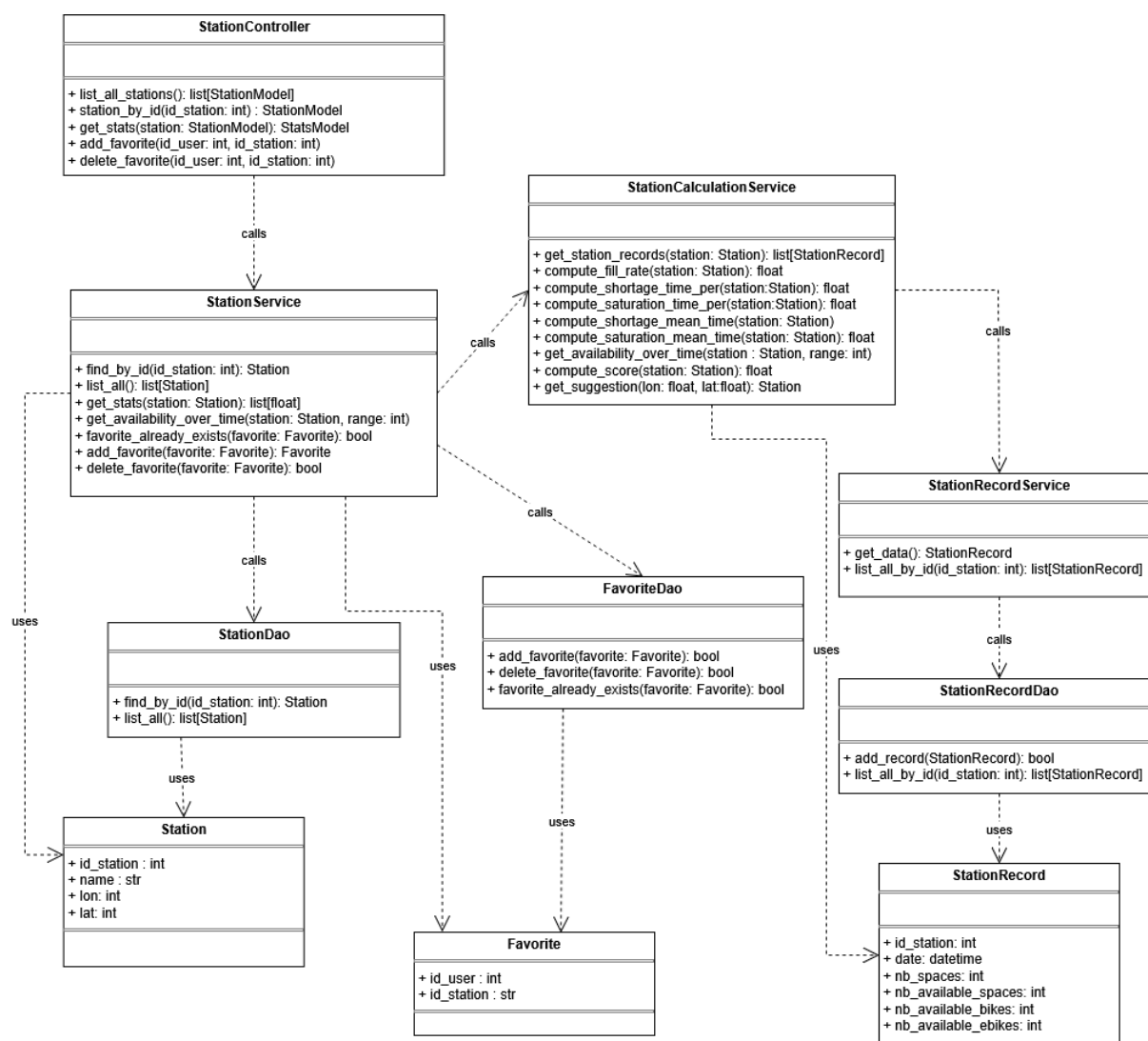
Figure 5: Diagramme de classes lié aux stations
