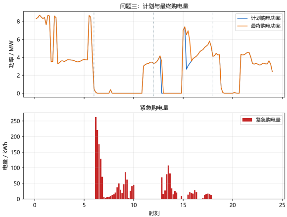
图 11: 计划量、最终购电量与紧急购电量的日内剖面（虚线为三个调整时刻）
