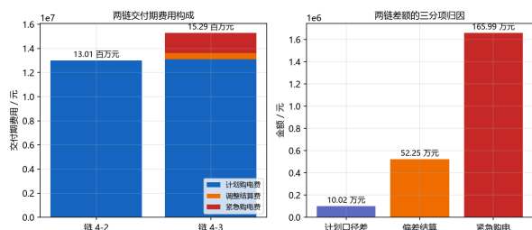
图 14：两链费用分项与交付期差额的三分项分解
