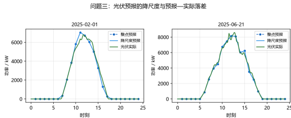
图 10: 光伏预报的降尺度与“预报—实际”落差
