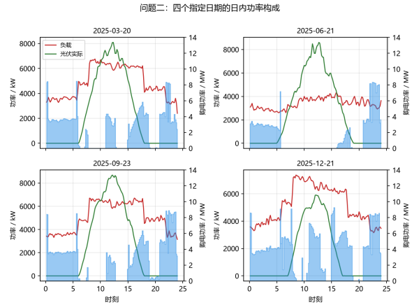
图 7: 题面四个指定日期的日内功率构成
