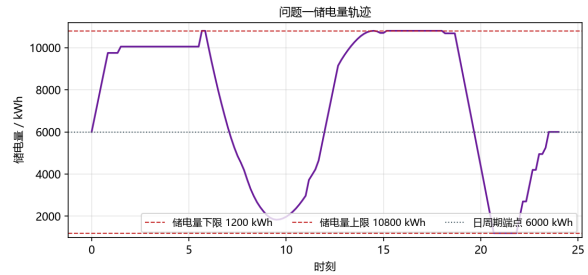
图 5：问题一储能电量轨迹
