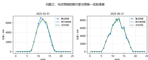
图 10: 光伏预报的降尺度与“预报—实际”落差
