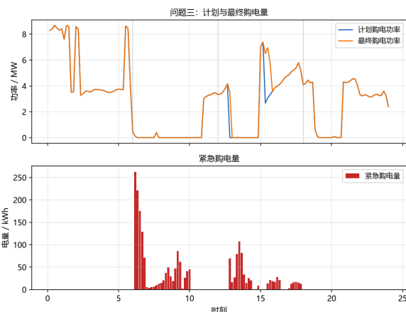
图 11: 计划量、最终购电量与紧急购电量的日内剖面（虚线为三个调整时刻）
