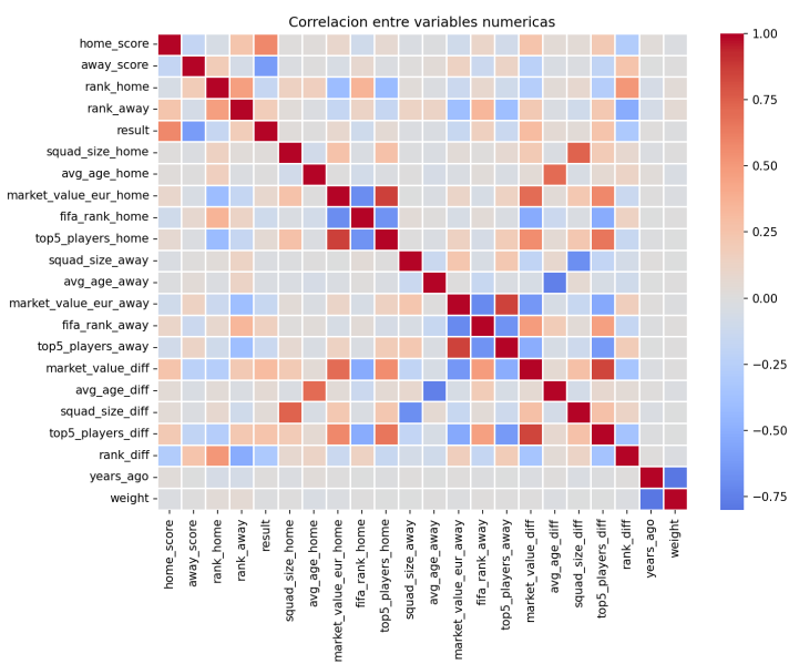
Figura 3. Heatmap de correlación entre variables
