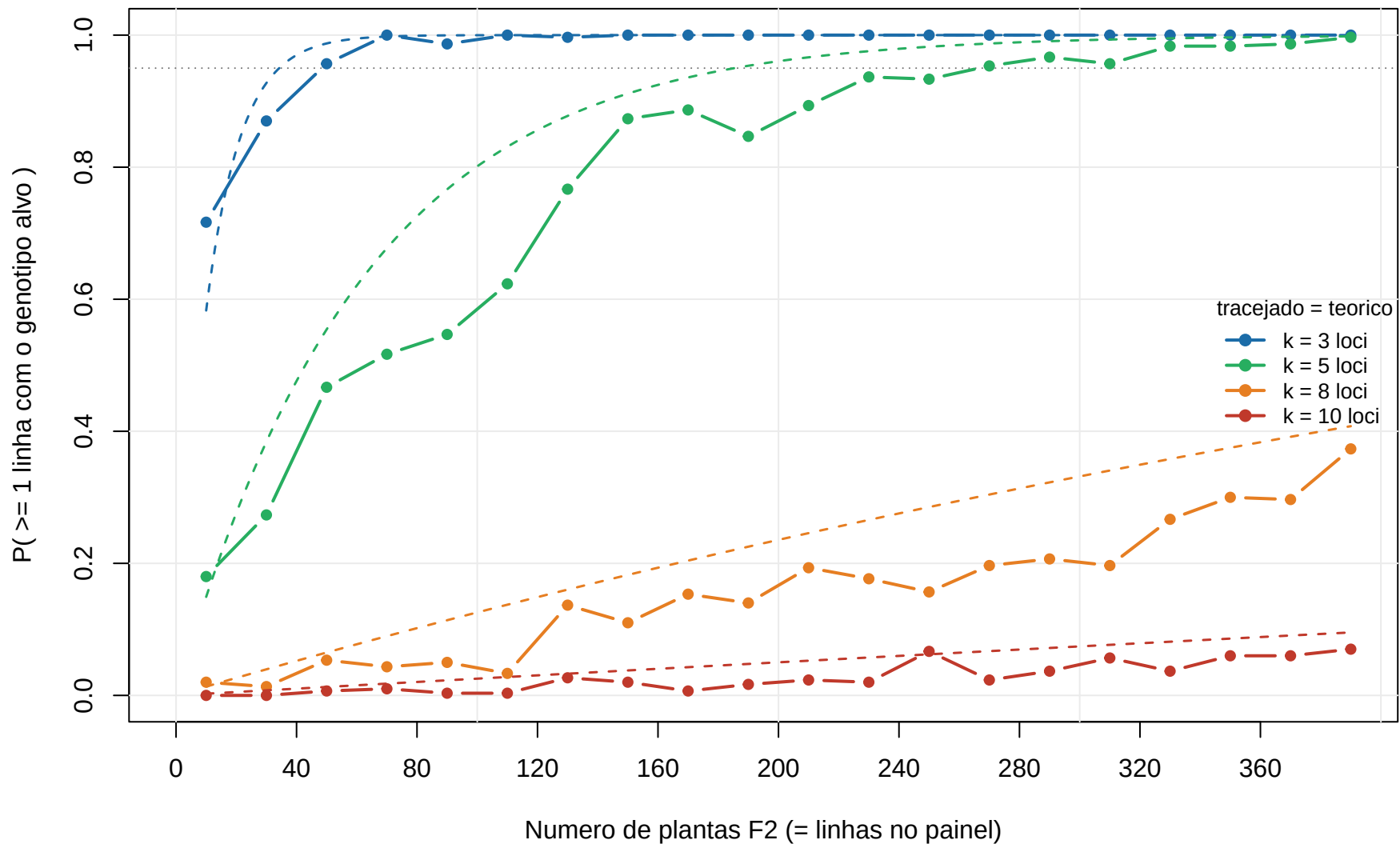
Fig 6. Recuperacao de combinacoes multilocus
