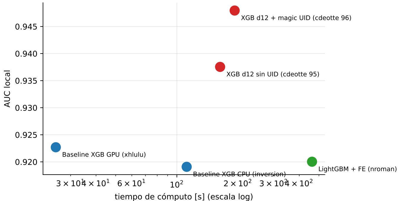
Precisión vs costo computacional (16 cores CPU / RTX 2060 6 GB)
