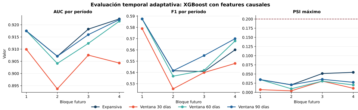
Figura 4.2: Evolución de AUC, F1 y PSI por bloque. El descenso del segundo bloque muestra que el rendimiento puede degradarse aunque el drift distributivo no supere el umbral alto de PSI; por ello se monitorean también métricas de desempeño.
