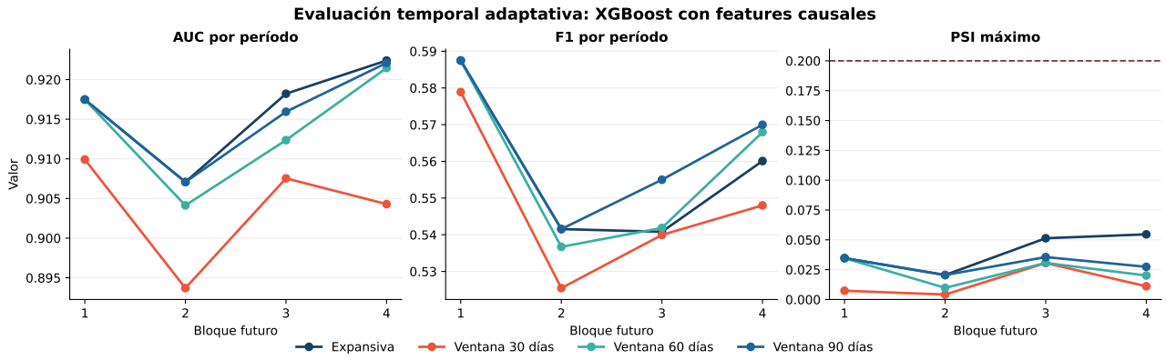
Figura 2: Evolución temporal de AUC, F1 y PSI. El segundo bloque muestra una degradación del modelo expansivo, aunque el PSI no supera el umbral alto.
