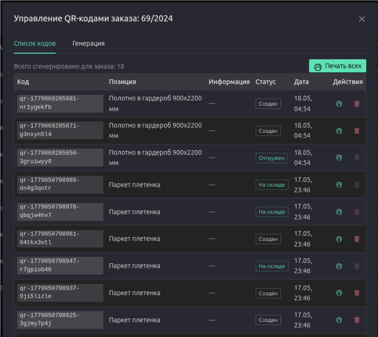
Рисунок 8 — Модальное окно управления QR-кодами заказа
