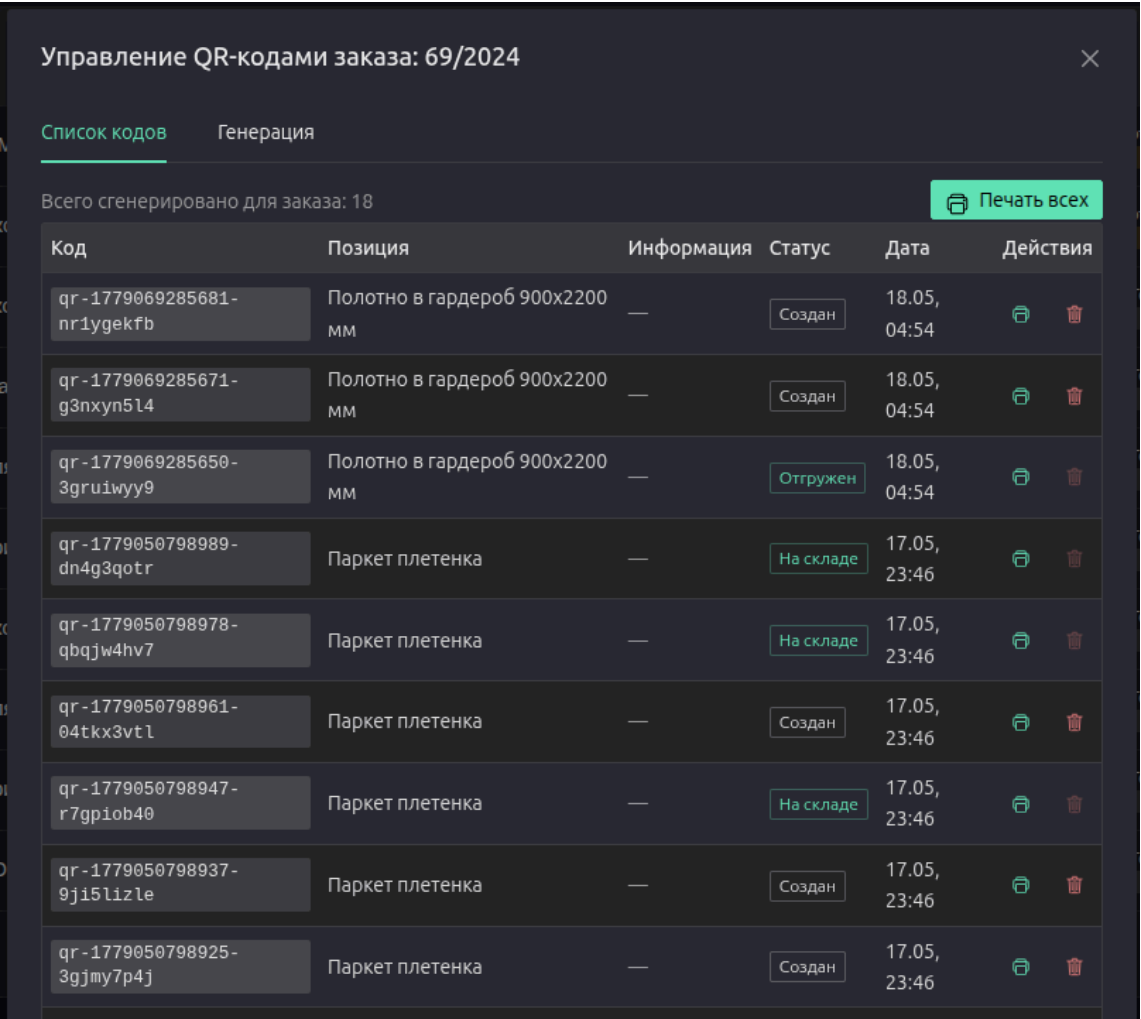
Рисунок 12 — Модальное окно управления QR-кодами заказа
