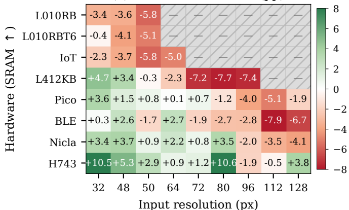
(a) VWW: \Delta TFLite acc. (pp)
