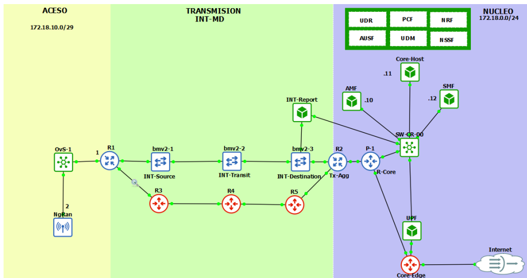
Figure 6.17: Diagrama de red para comparación de latencias en N3
