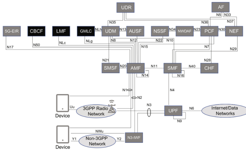
Figure 2.3: Arquitectura 5GC con interfaces punto a punto. [4].
