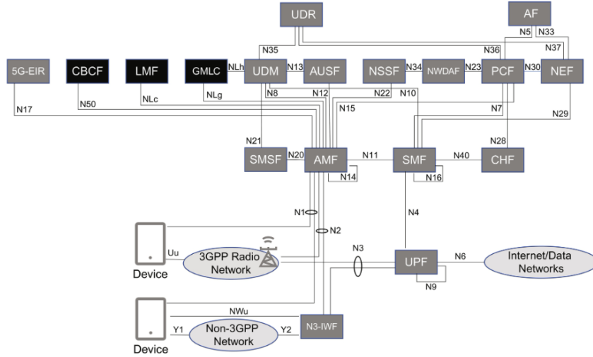
Figura 2.3: Arquitectura 5GC con interfaces punto a punto. [18].
