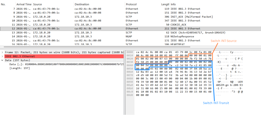
Figure 6.6: Captura de paquetes INT enviado a INT-Sink
