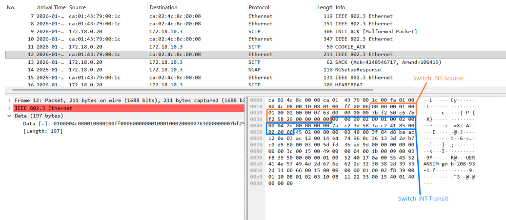
Figure 6.6: Captura de paquetes INT enviado a INT-Sink
