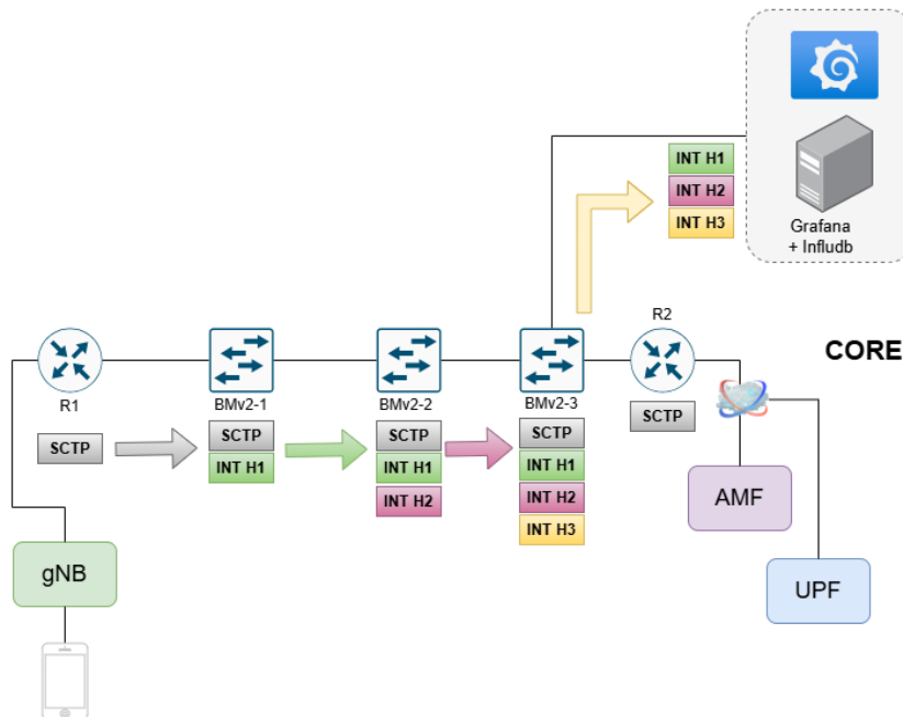
Figura 4.20: Topología INT-MD
