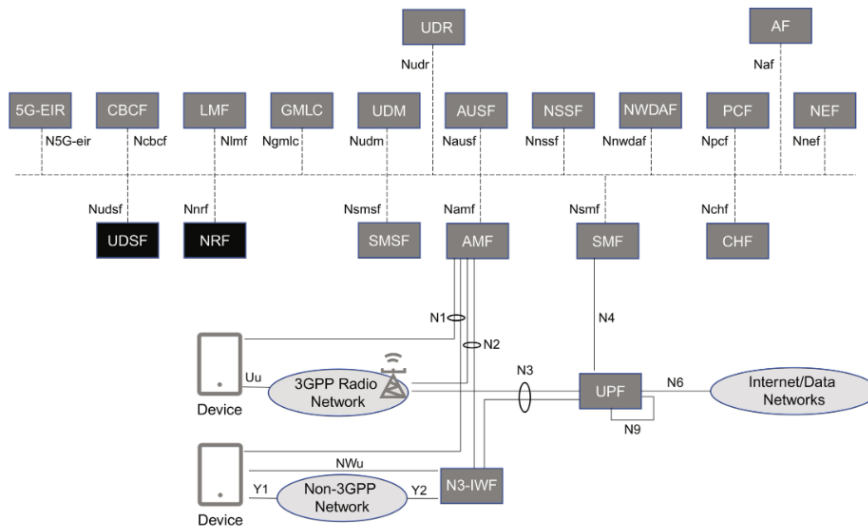
Figura 2.2: Arquitectura 5GC basada en interfaces basadas en servicios [18].
