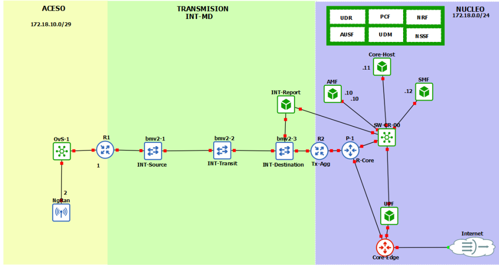
Figura 4.2: Topología de red implementada en GNS3
