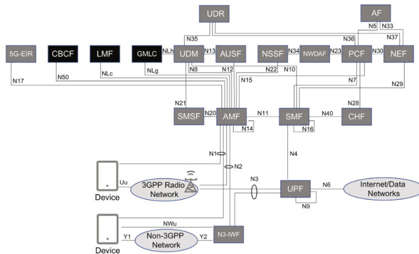
Figura 2.3: Arquitectura 5GC con interfaces punto a punto. [18].
