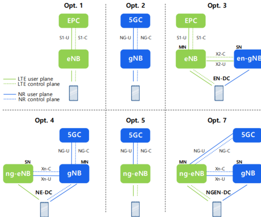
Figura 2.1: Opciones de implementación de NR en 5G: NSA y SA [3].
