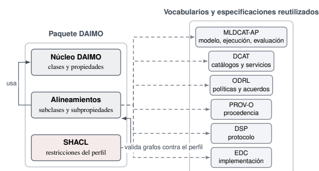
Figura 1. Organización modular del paquete DAIMO y recursos reutilizados.
