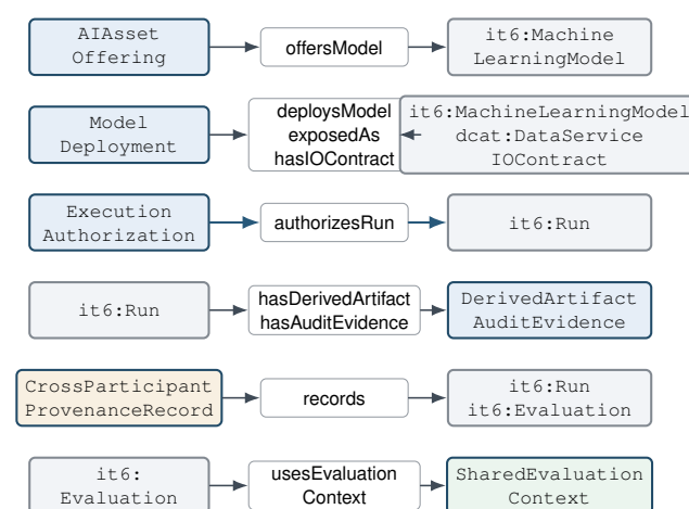
Figura 3. Alineamientos externos y relaciones principales de DAIMO.
