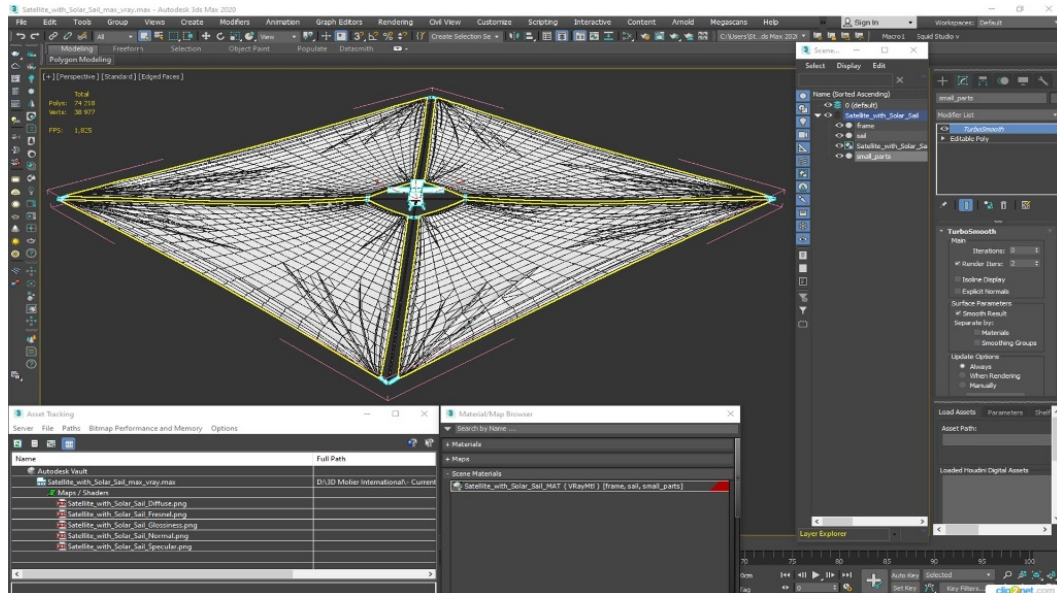
Figura 2.5: Visualizzazione wireframe (a fil di ferro) della membrana solare simulata. La suddivisione in triangoli permette di calcolare la spinta fotonica in modo dettagliato su tutta la superficie.
