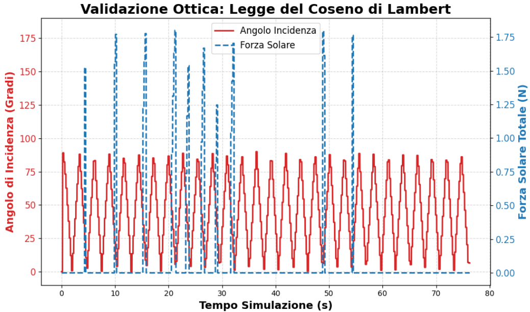
Figura 6.2: Correlazione tra l'angolo di incidenza dei fotoni e l'intensità della forza solare risultante.
