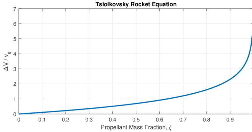
Figura 1.1: Andamento del rapporto tra variazione di velocità e velocità di scarico ( \Delta v/v_e ) in funzione della frazione di massa del propellente ( \zeta ).
