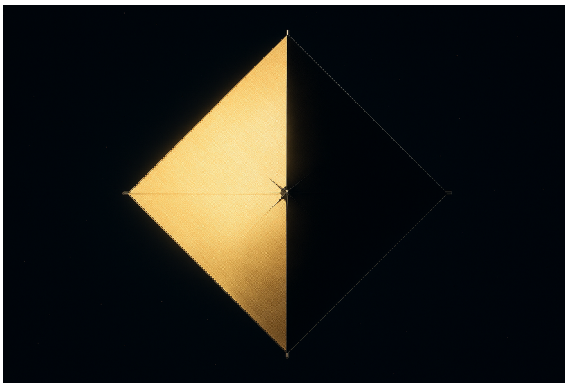
Figura 1.6: Effetto dell'occlusione ambientale parziale: l'asimmetria di illuminazione sposta il centro di pressione rispetto al centro di massa, generando un momento torcente ( torque ) che induce il rotolamento del veicolo.
