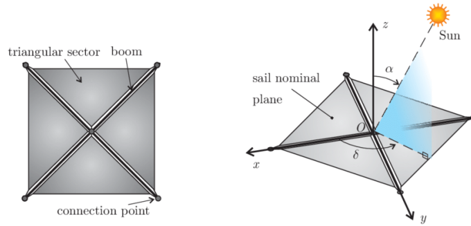
Figura 1.4: Astrazione vettoriale dell'interazione fotonica. L'angolo \alpha , compreso tra la normale del piano nominale e la direzione del Sole, governa la riduzione geometrica dell'area utile ai fini propulsivi.
