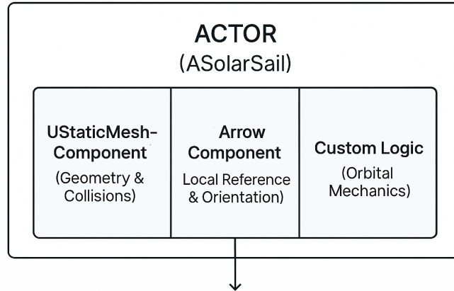
Figura 2.1: Architettura del paradigma Actor-Component : l'Attore agisce da contenitore unificatore per le logiche visive, fisiche e di collisione.
