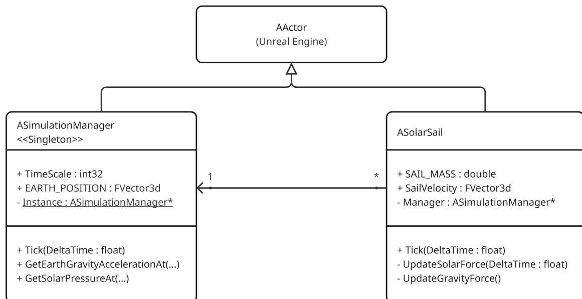
Figura 2.3: Diagramma UML semplificato che mostra l'ereditarietà dalla classe AActor di Unreal Engine e le relazioni tra le classi principali del simulatore.
