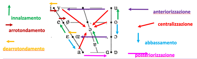
FIGURA 1: Trapezio vocalico
