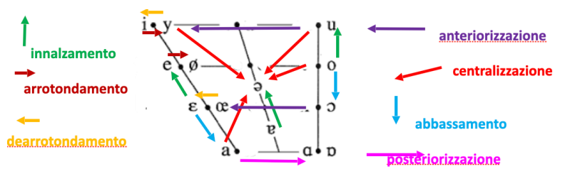
FIGURA 1: Trapezio vocalico
